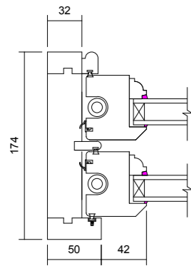
03 Jamb Detail 1 : 5
