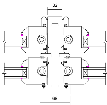
04 Mullion Detail 1 : 5
