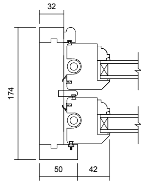
03 Jamb Detail 1 : 5
