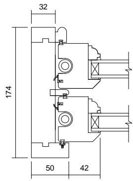
03 Jamb Detail 1 : 5
