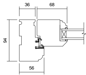
03 Jamb Detail 1:5
