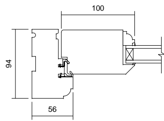
03 Jamb Detail 1 : 5
