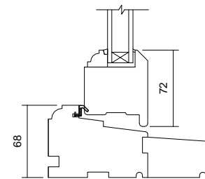
06 Transom Detail 1 : 5
