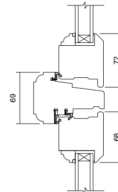
06 Transom Detail 1 : 5
