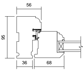
03 Jamb Detail 1 : 5
