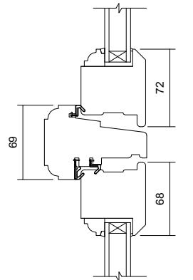
06 Transom Detail 1 : 5
