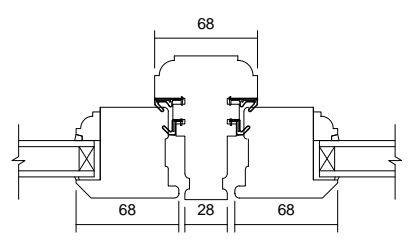
04 Mullion Detail 1 : 5
