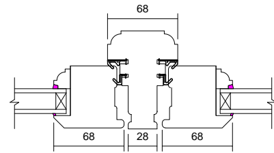
7 Mullion Detail 1 : 5
