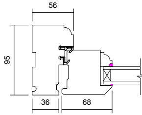
03 Jamb Detail 1 : 5
