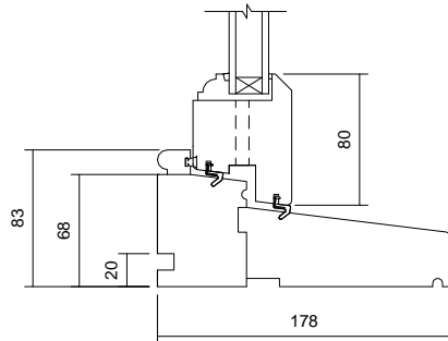
07 Sill Detail 1 : 5
