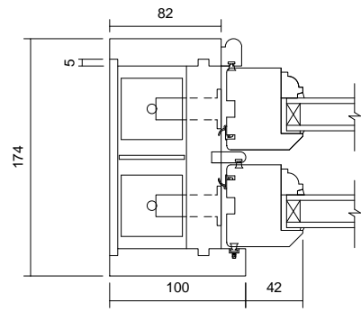
03 Jamb Detail 1 : 5
