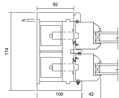
03 Jamb Detail 1 : 5
