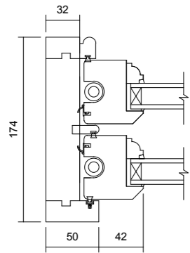
03 Jamb Detail 1 : 5
