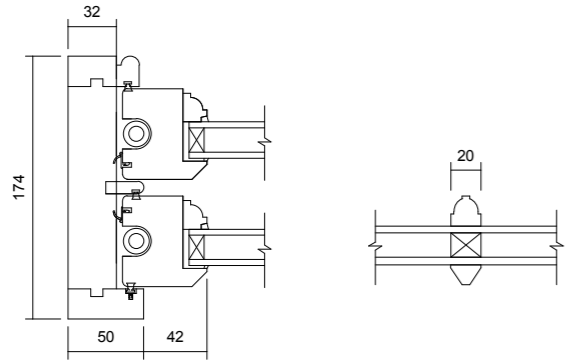
03 Jamb Detail 1 : 5
