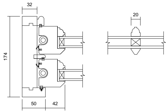
03 Jamb Detail 1 : 5
