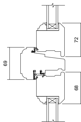
06 Transom Detail 1 : 5
