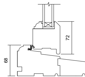
08 Cill Detail 1 : 5
