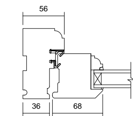
03 Jamb Detail 1 : 5
