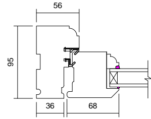
03 Jamb Detail 1 : 5
